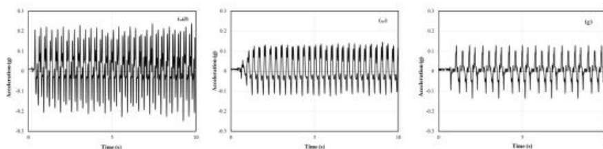
شکل ۴. نمونه‌ای از تاریخچه‌های زمانی شتاب در فرکانس ۳ هرتز و شتاب ورودی ۰/۱g در شتاب‌سنج A_2 تحت بارگذاری الف) مستطیلی، ب) سینوسی و ج) مثلثی
