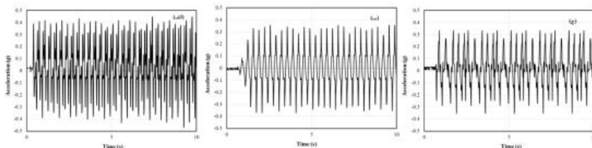
شکل ۵. نمونه‌ای از تاریخچه‌های زمانی شتاب در فرکانس ۳ هرتز و شتاب ورودی ۰/۳g در شتاب‌سنج A_2 تحت بارگذاری الف) مستطیلی، ب) سینوسی و ج) مثلثی
