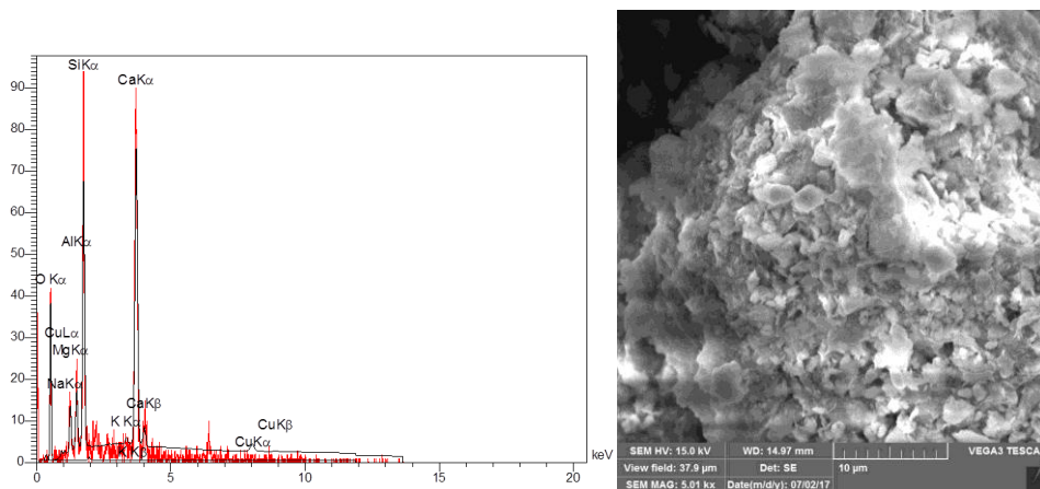
شکل ۱۰. الف). تصویر میکروسکوپ الکترونی پویشی از نمونه خاک مارن تثبیت شده با ۰.۴٪ سیمان و ۱٪ نانوسیلیس پس از ۲۸ روز عمل‌آوری، ب) طیف‌سنجی پاشندگی انرژی (EDS) از نمونه مارن تثبیت شده با ۰.۴٪ سیمان و ۱٪ نانوسیلیس پس از ۲۸ روز عمل‌آوری
