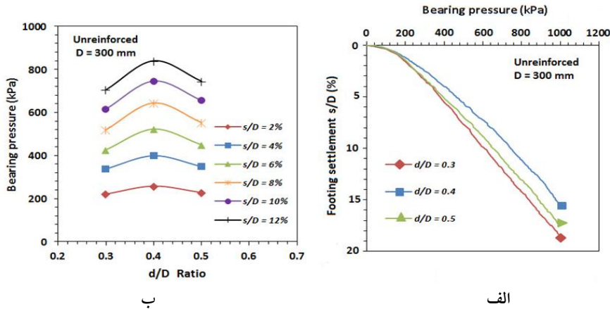
شکل ۶. نمودار تغییرات ظرفیت باربری پی رینگ مستقر بر بستر غیرمسلح در برابر الف) نسبت نشست ( s/D )، ب) نسبت قطر داخلی به خارجی پی رینگ ( d/D )
