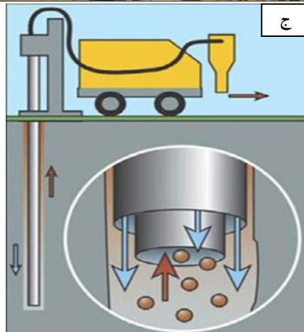
شکل ۱. الف) نمای از عملیات حفاری به روش RC در معدن طلای اخترچی خمین، ب) نمایی نزدیک از سیکلون دستگاه حفاری RC، ج) شکل طرح وار از سیستم نمونه‌گیری به وسیله روش RC [۴]
