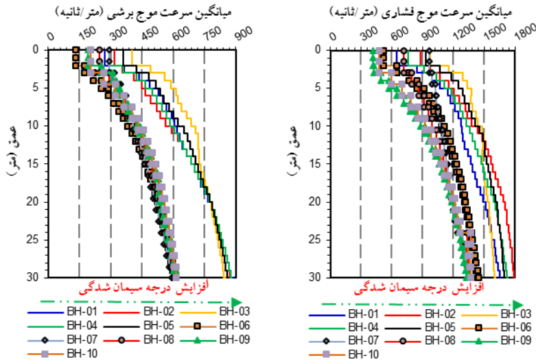
شکل ۱۴. نتایج آزمون‌های لرزه‌ای درون‌گمانه‌ای، الف) میانگین سرعت موج برشی، ب) میانگین سرعت موج فشاری
