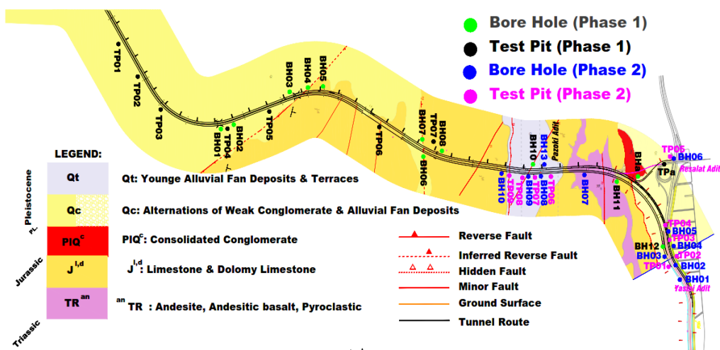
شکل ۱. الف) نقشه زمین‌شناسی و گسل‌های شهر تهران، ب) پلان زمین‌شناسی و موقعیت گمانه‌ها و چاهک‌های شناسایی مسیر تونل [۲۱]
