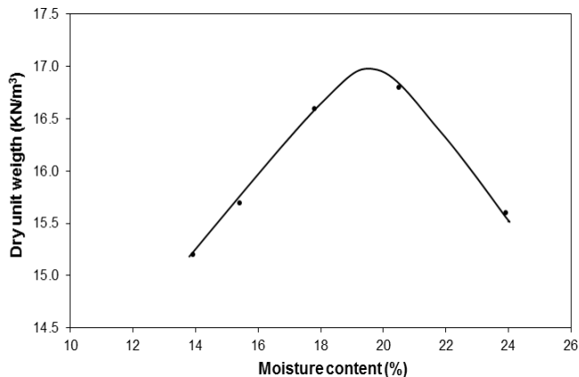
شکل ۲. نمودار تراکم خاک پایه به روش تراکم استاندارد یا پروکتور (ASTM D698)
