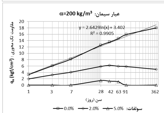
شکل ۵. تأثیر تغییر عیار سیمان ضد سولفات تیپ ۵ و درصد سولفات سدیم بر مقاومت فشاری تک محوری نمونه‌ها با عیار سیمان الف) ( 400 \text{ kg/m}^3 )، ب) ( 300 \text{ kg/m}^3 )، ج) ( 200 \text{ kg/m}^3 )
