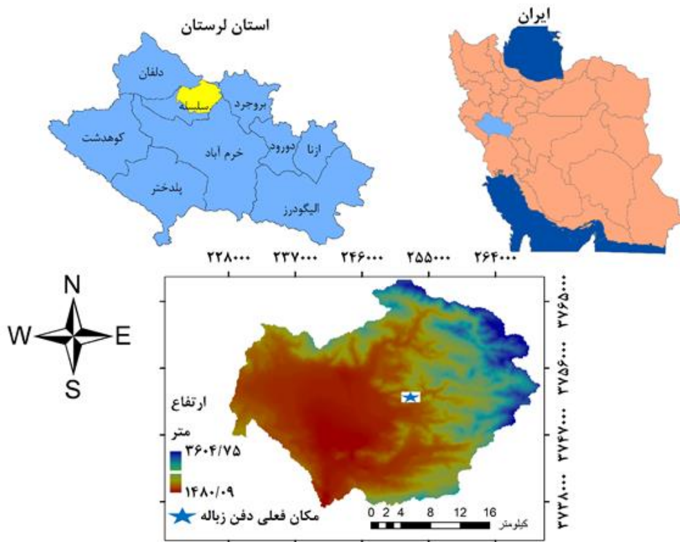
شکل ۱: موقعیت منطقه مورد مطالعه در استان لرستان و ایران
