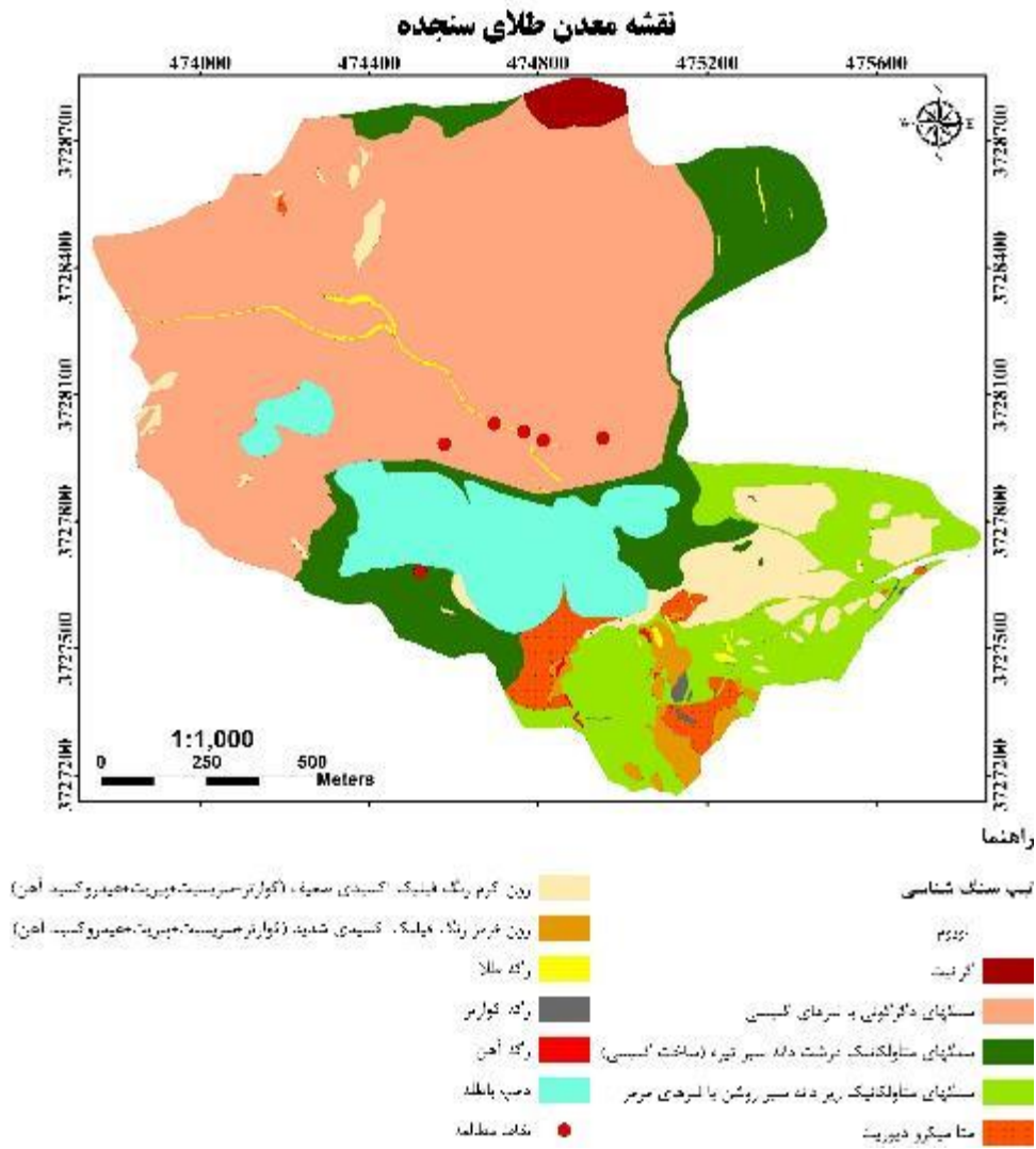
شکل شماره ۲- نقشه زمین شناسی معدن سنجهده و محل نمونه گیری در شیست هایی که در دیواره معدن مشکل ایجاد نموده اند [۲۳]
