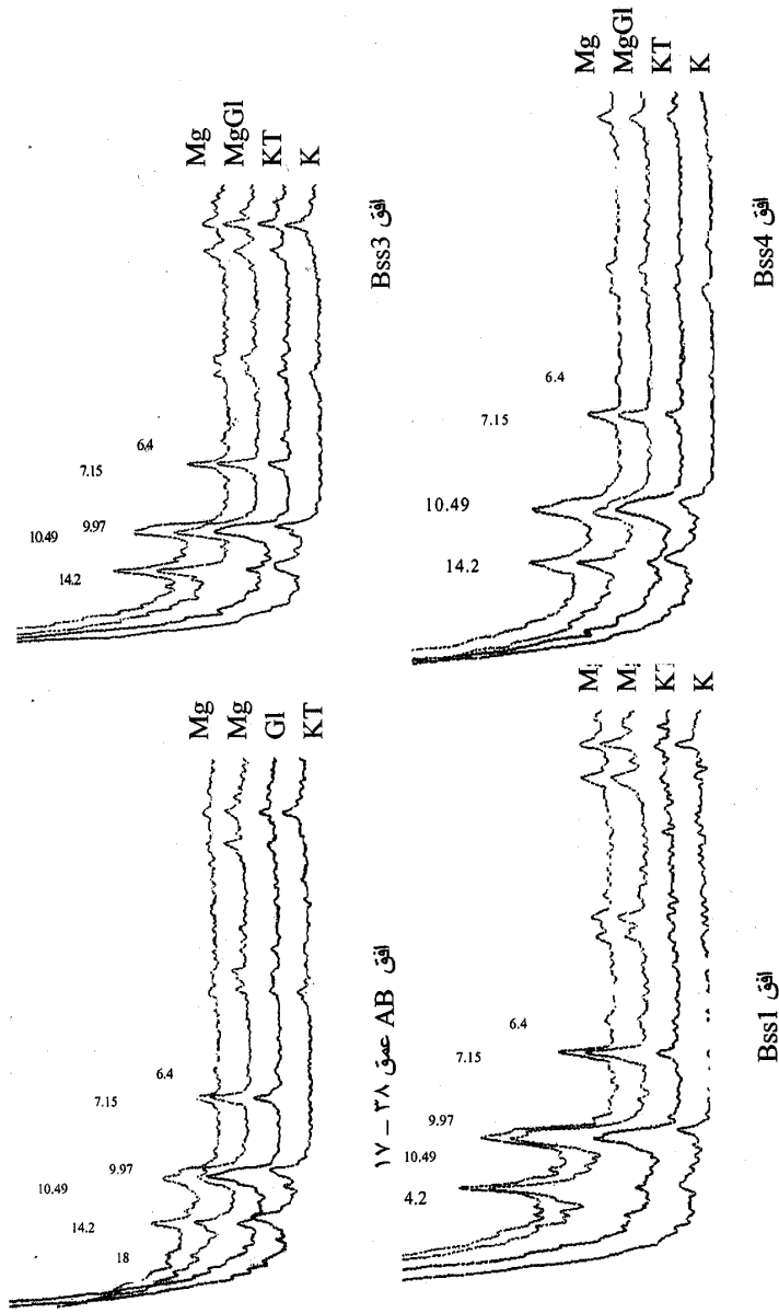
شکل ۲- دیفرکتوگرام های رس کل پروفیل شماره ۴
