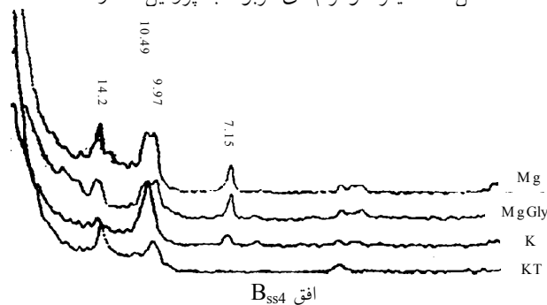
شکل ۶ - دیفراکتوگرام مربوط به پروفیل شماره ۷
