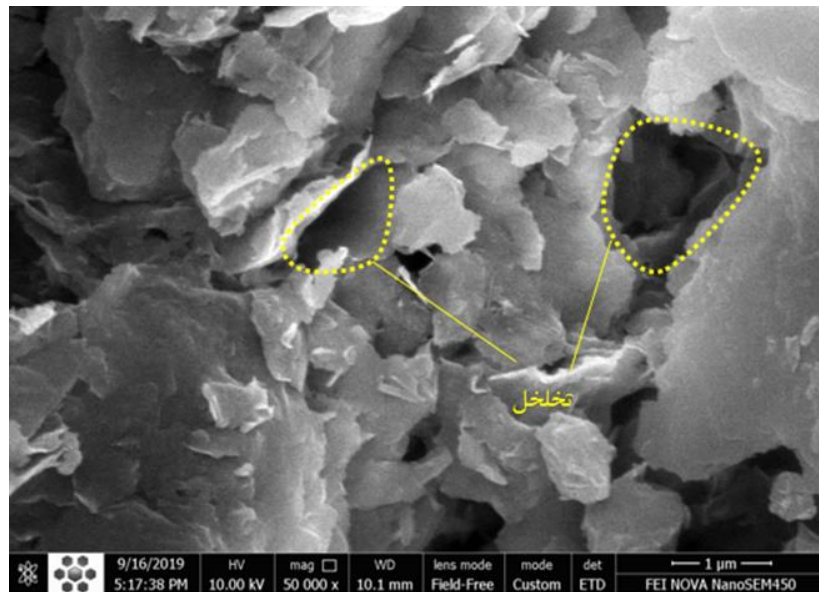
شکل ۲۱- خاک مارن مورد مطالعه تثبیت شده با پنج درصد سیمان
