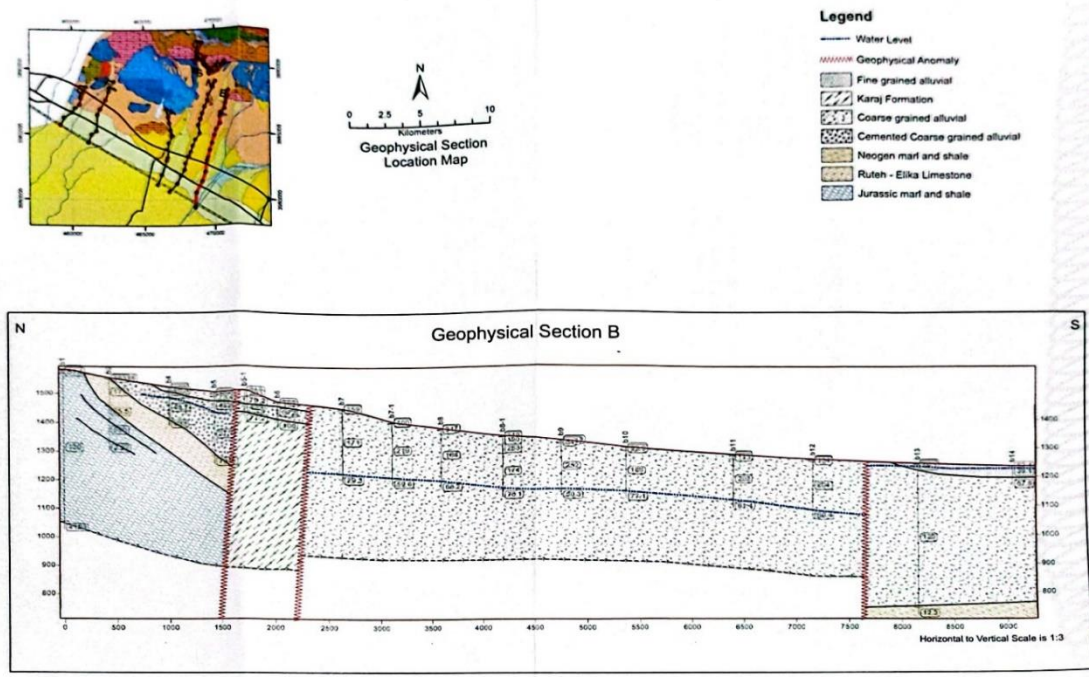
شکل ۱۲. مقطع ژئوفیزیکی B Fig. 12. Geophysical cross section B
