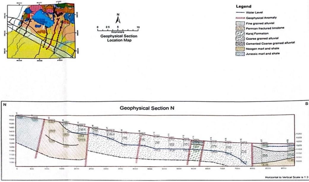
شکل ۱۱. مقطع ژئوفیزیکی N Fig. 11. Geophysical cross section N
