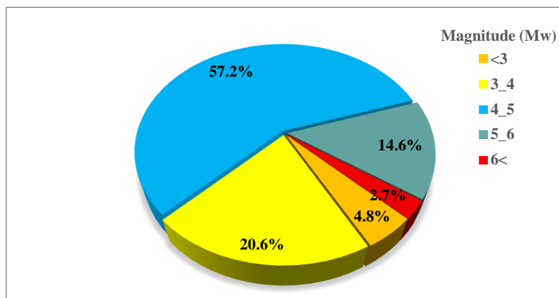
شکل ۴. فراوانی زمین‌لرزه‌ها در بازه‌های مختلف بزرگی در پیرامون ساختگاه (بازه زمانی ۱۹۰۰ تا ۲۰۲۲)
