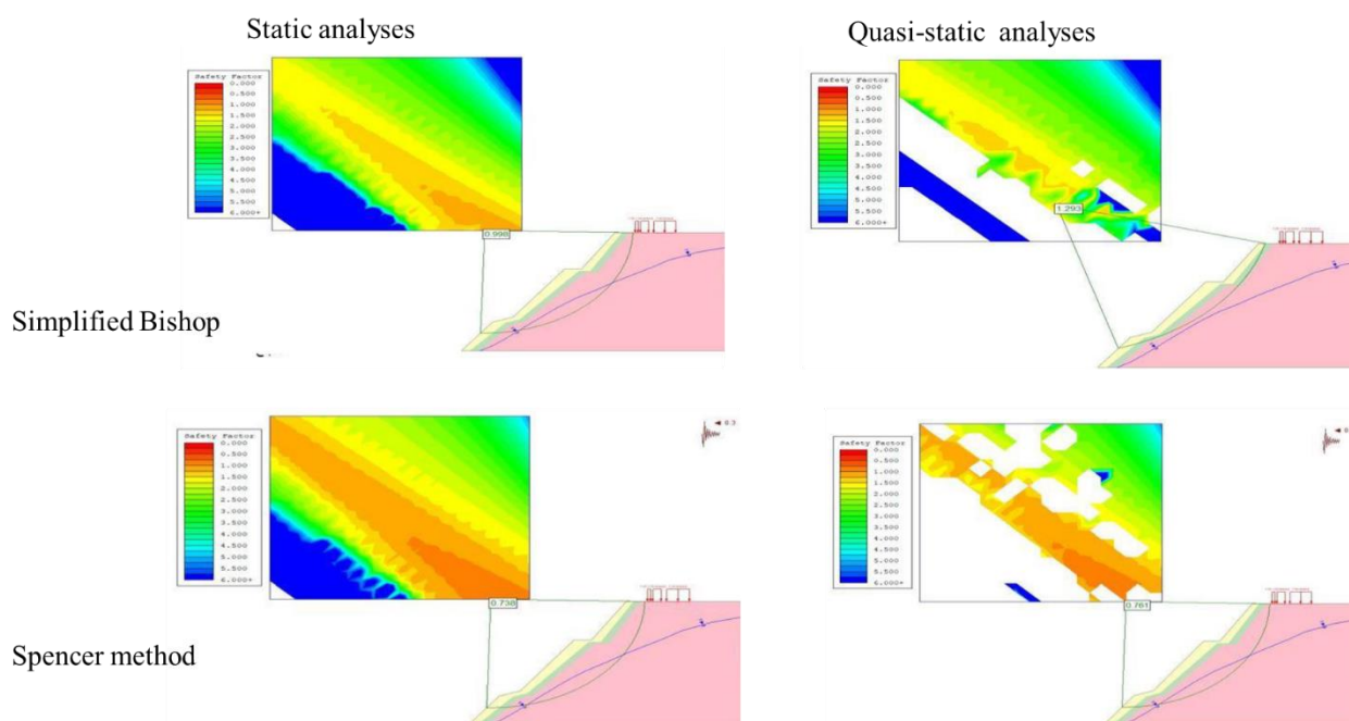
شکل ۱۲. نتایج تحلیل پایداری نرم افزار اسلاید در شرایط اشباع برای پروفیل B
