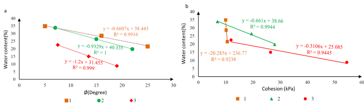
شکل ۷. تأثیر افزایش درصد رطوبت در کاهش (a) زاویه اصطکاک داخلی و (b) چسبندگی در پروفیل‌های مورد مطالعه Fig. 7. The effect of increasing moisture percentage on the reduction of a: internal friction angle and b: cohesion in the studied profiles
