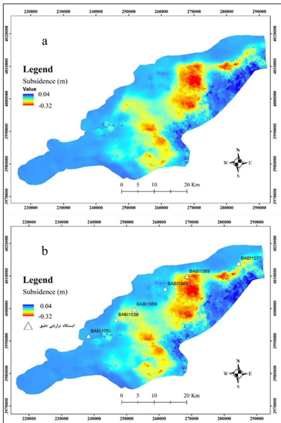
شکل ۵. ا) نقشه پهنه‌بندی نهایی فرونشست زمین در آبخوان دامغان با بیشینه نرخ حدود ۳۲ سانتی‌متر؛ ب) مقایسه نرخ فرونشست سالانه در ایستگاه BABI ۱۰۶۹ بین داده‌های InSAR و ترازبایی دقیق Fig. 5. a) Final land subsidence zoning map of the Damghan plain with a maximum rate of approximately 32 cm; b) Comparison of annual subsidence rates at station 1069BABI based on InSAR and precise leveling data.
