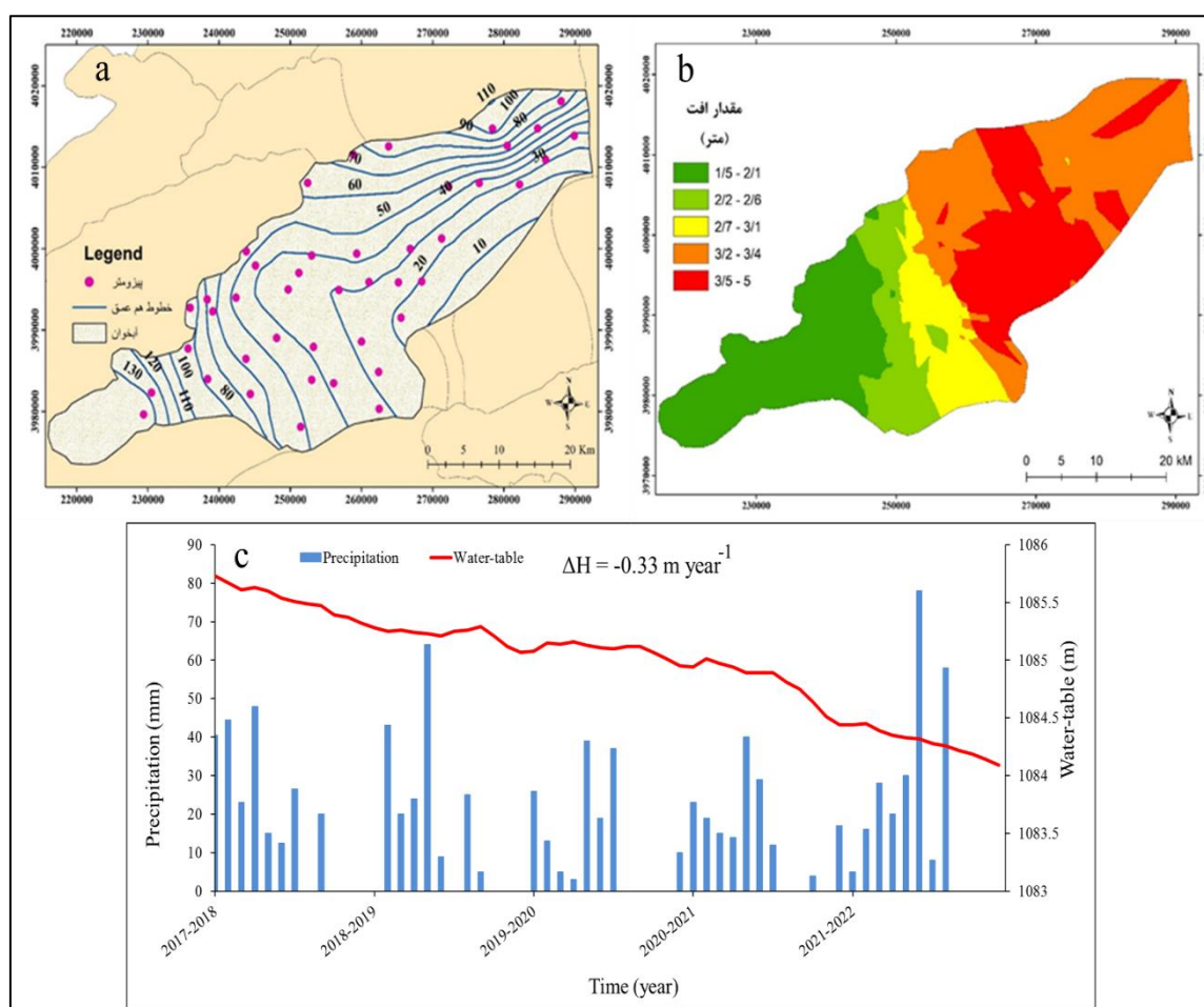
شکل ۳- ا) تغییرات عمق آب زیرزمینی در آبخوان دامغان؛ ب) مقادیر افت آب زیرزمینی در آبخوان دامغان؛ ج) هیدروگراف معرف آبخوان دامغان. Fig. 3. a) Groundwater depth variations; b) Decline values; c) Representative hydrograph of the Damghan aquifer.
