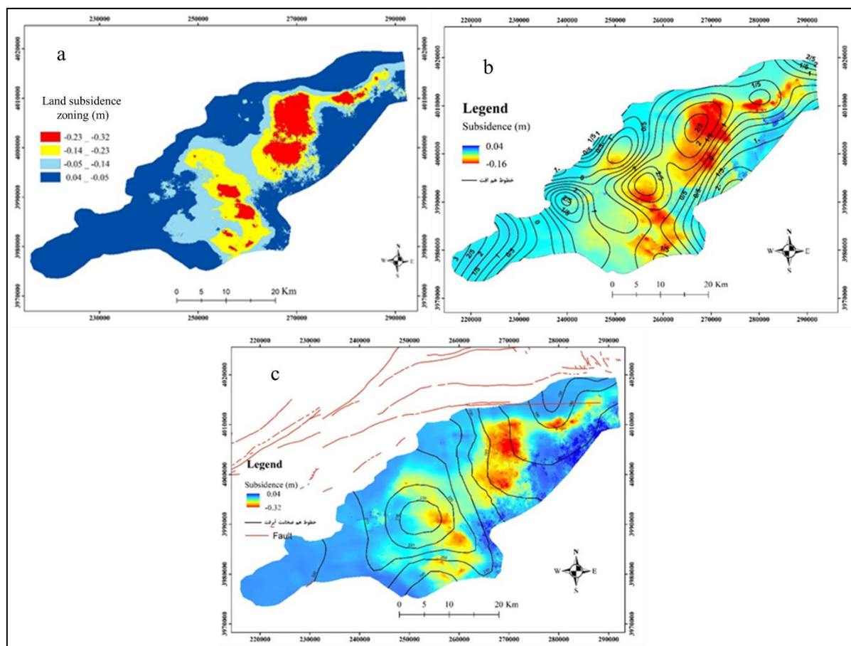
شکل ۷-۷) زون‌بندی نرخ متوسط فرونشست زمین در آبخوان دامغان طی سال‌های ۲۰۱۷ تا ۲۰۱۹؛ (b) هم‌پوشانی افت سطح آب زیرزمینی با نواحی دارای نرخ بالای فرونشست؛ (c) عدم ارتباط معنادار میان موقعیت گسل‌ها و محدوده فرونشست.
