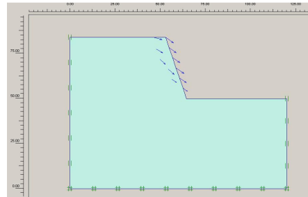
شکل ۳. نمایش تغییرشکل‌های کل برای تحلیل دوبعدی برای تراشه با ارتفاع ۳۴ متر، شیب ۱ افقی: ۲ قائم و مصالح L1-1
