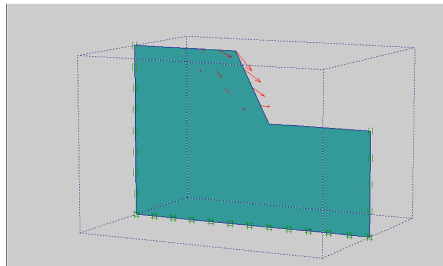
شکل ۳. نمایش تغییرشکل‌های کل برای تحلیل دوبعدی برای تراشه با ارتفاع ۳۴ متر، شیب ۱ افقی: ۲ قائم و مصالح L1-1
