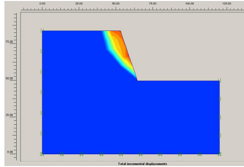
شکل ۳. نمایش تغییرشکل‌های کل برای تحلیل دوبعدی برای تراشه با ارتفاع ۳۴ متر، شیب ۱ افقی: ۲ قائم و مصالح L1-1
