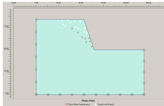
شکل ۵. نقاط پلاستیک شده و تحت کشش در حالت دوبعدی برای تراشه به ارتفاع ۳۴ متر با شیب ۱ افقی: ۲ قائم و مصالح L1-1
