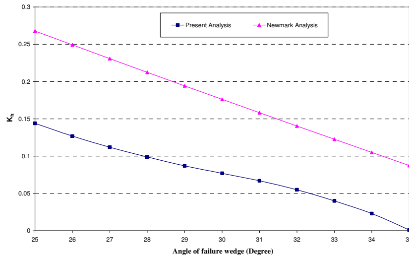
شکل ۹. تغییرات ضریب شتاب لرزه‌ای افقی تسلیم در برابر زاویه گسختگی
