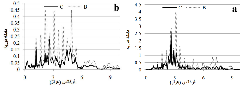
شکل ۱۱. طیف دامنه فوری برای بالاترین عمل کرد RSM (در عمق ۱۰ متری سنگ‌بستر) در اثر شتاب‌نگاشت قوی (a) و ضعیف (b)
