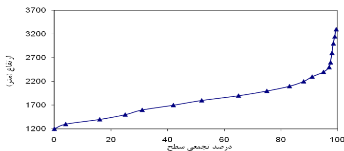
شکل ۱۰. منحنی ارتفاع-سطح حوزهٔ آبریز گاماسیاب پایین
