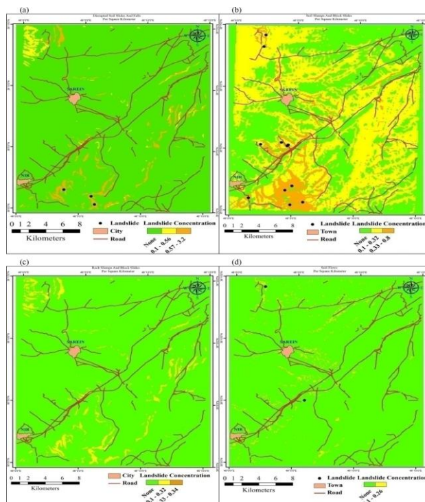
شکل ۱۳. تراکم خطر زمین‌لغزش‌های ناشی از زلزله محاسبه شده برای زلزله ۱۳۷۵ سرعین، اردبیل با M_w = 6.1 (a) تراکم‌های پیش‌بینی شده ریزش‌ها و لغزش‌های خاکی گسسته با استفاده از کامل، (b) تراکم‌های پیش‌بینی شده لغزش‌های بلوکی و چرخشی خاکی با استفاده از کامل، (c) تراکم‌های پیش‌بینی شده لغزش‌های بلوکی و چرخشی سنگی با استفاده از کامل، (d) تراکم‌های پیش‌بینی شده جریان‌های خاکی سریع با استفاده از کامل. دایره‌های توپر زمین‌لغزش‌های رخ داده ناشی از زلزله ۱۳۷۵ سرعین، اردبیل هستند.
