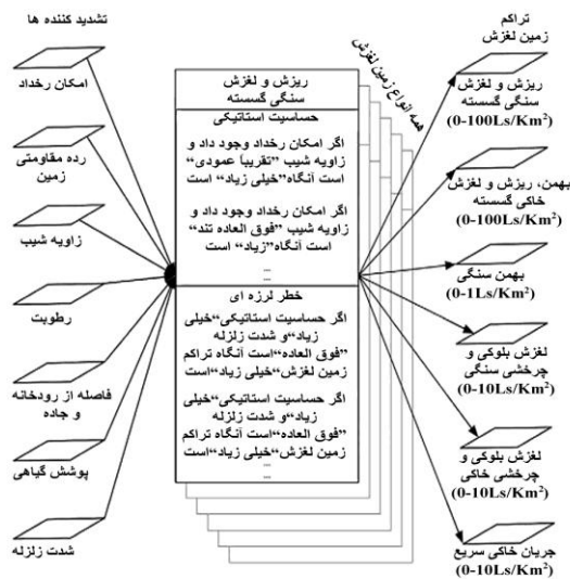
شکل ۱۱. نمودار جریانی داده‌ها برای بخش مقدار تراکم خطر کامل، معرف ورودی‌ها (اطلاعات تشدید کننده)، خروجی‌ها، و ترتیب قواعد [۱۱]، [۱۲]
