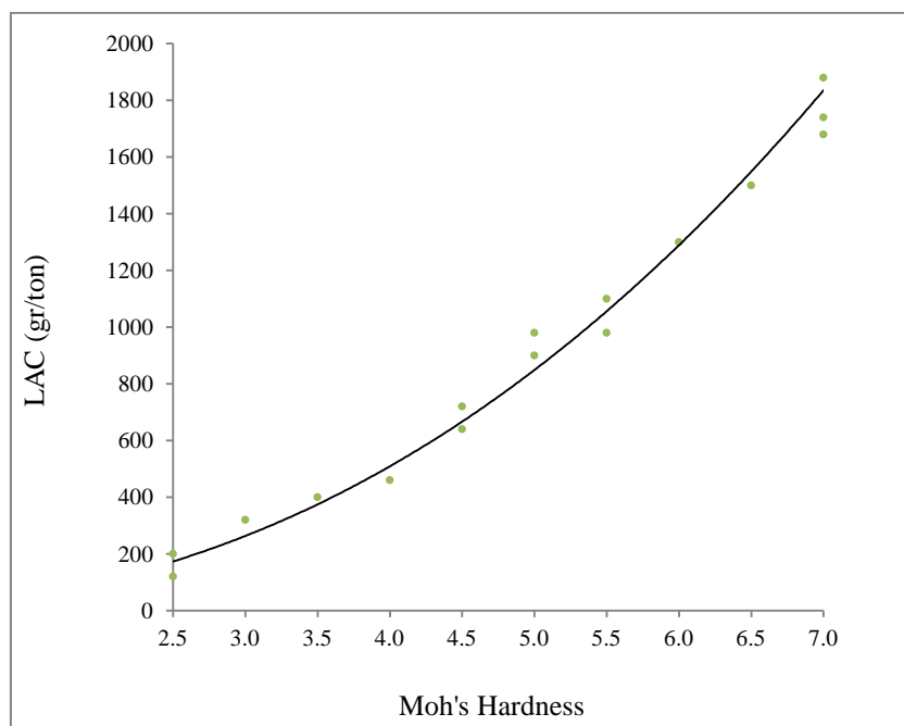
شکل ۶. محدوده مقادیر LAC در برابر سختی موس
