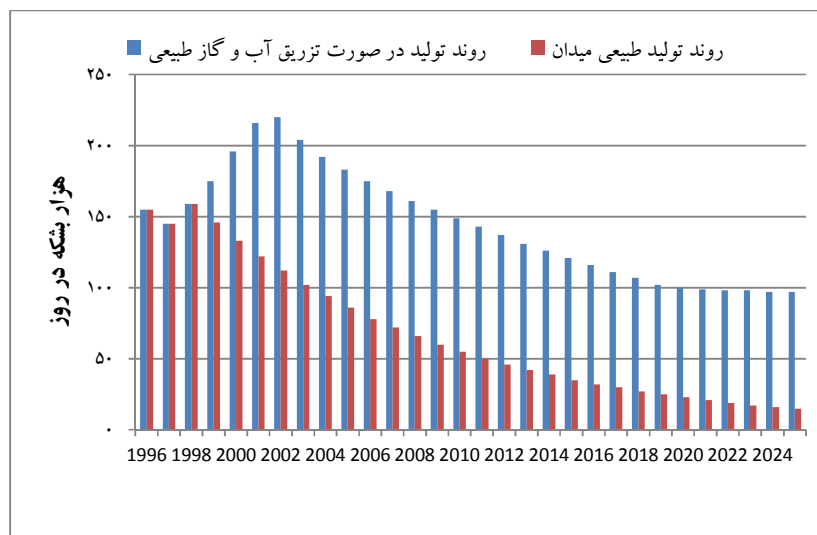
نمودار ۱. پیش بینی نرخ تولید روزانه نفت خام در دو گزینه برداشت اولیه و ثانویه
