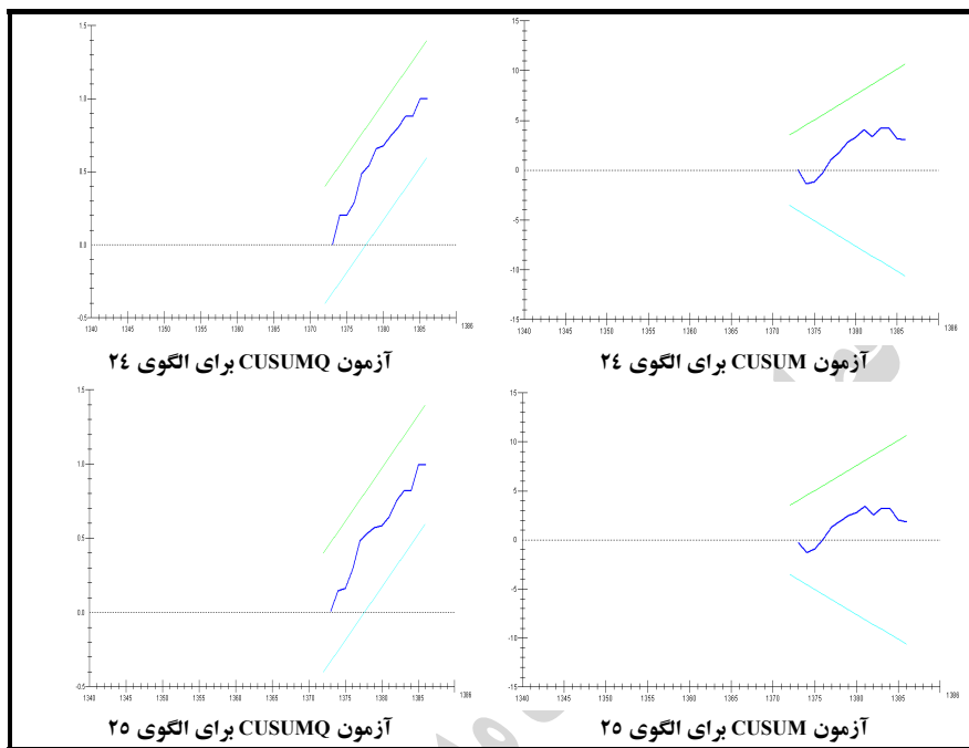
شکل ۱. آزمون‌های ثبات ضرایب CUSUM و CUSUMQ
