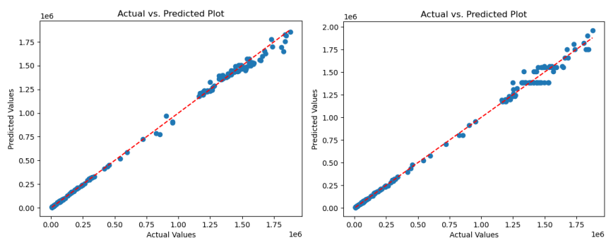
شکل ۵. نمودار پراکندگی RF
