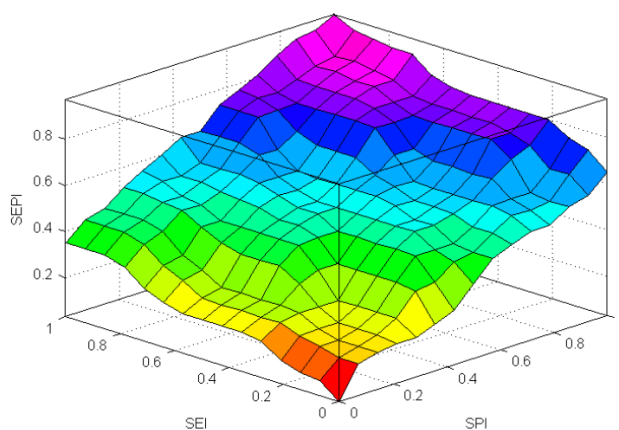
شکل (۵) نمایشی از Surface Viewer در محیط MATLAB
