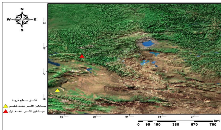
شکل (۳). موقعیت استقرار هسته سامانه پرفشار سیبری در ماه اکتبر در دهه اول و ششم دوره آماری (۱۹۵۵-۲۰۱۴)
