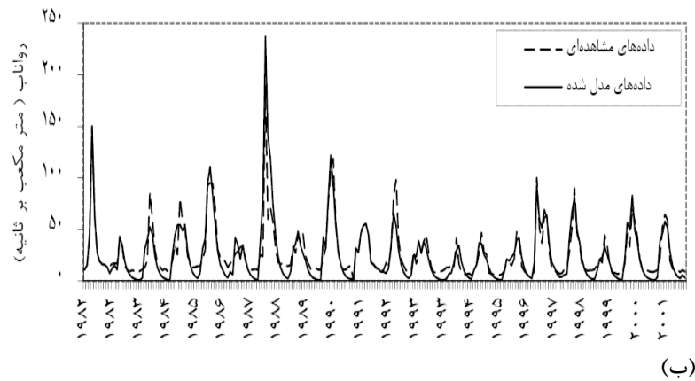
شکل (۵) مقایسه رواناب مشاهداتی حوضه با رواناب مدل شده توسط IHACRES در دوره (الف) و (ب) و اسنجی (ب) و صحت سنجی
