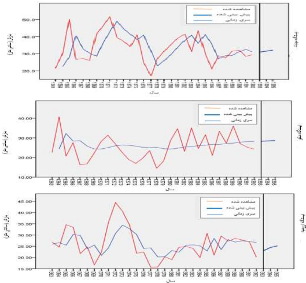
شکل (۶). نمودار مقادیر پیش بینی شده و مشاهده ای برای داده های ایستگاه شده میانگین بارش سالانه بر اساس مدل مناسب در هر ایستگاه
