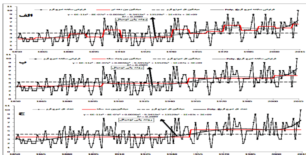
شکل (۷). روند نوسانات زمانی بین دهه‌ی (الف)، بین ۵۰ ساله (ب)، و بین ۱۰۰ ساله‌ی (ج) و پلکانی فراوانی وقوع امواج گرمایی در منطقه شمال غرب ایران در بازه زمانی ۱۸۵۰ تا ۲۰۱۴.
