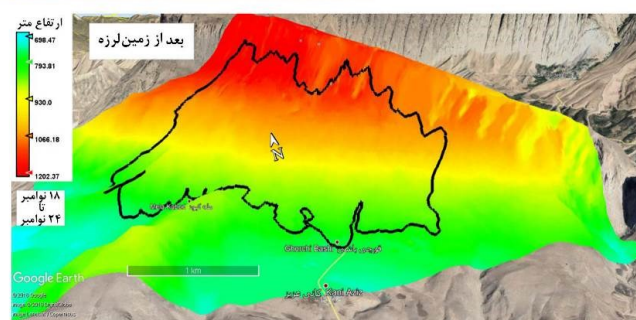
شکل (۶). همپوشانی مدل رقومی ارتفاعی حاصل از اینترفرومتری منطقه زمین لغزش مله کبود بر روی گوگل ارث
