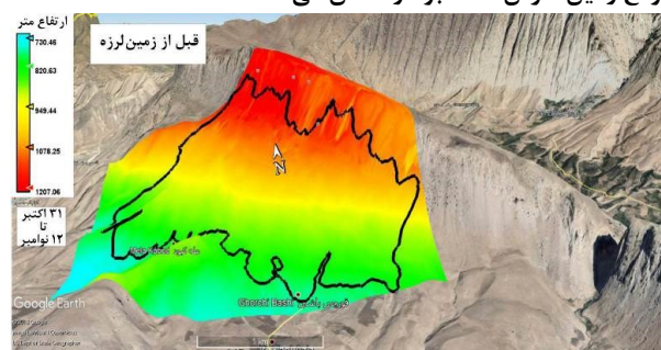
شکل (۵). مدل رقومی قبل (راست) و پس از زمین لرزه (چپ) از منطقه مورد مطالعه (تاریخ زمین لرزه ۱۲-۱۱-۲۰۱۷). پلی گون موقع زمین لغزش مله کبود را نشان می دهد.
