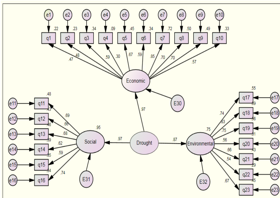
شکل (۳): مدل ساختاری تحلیل چهار عاملی تأییدی مرتبه دوم برای برآورد و تحلیل خشکسالی همراه با برآوردهای استاندارد مآخذ: یافته‌های تحقیق، ۱۳۹۷.
