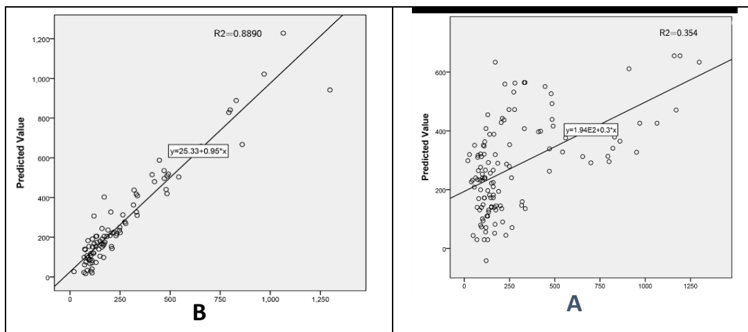
شکل (۶). نمودار پراکنندگی داده های واقعی و داده های پیش بینی شده توسط هر مدل، (a) مدل رگرسیون خطی چند متغیره، (b) مدل شبکه عصبی مصنوعی MLP
