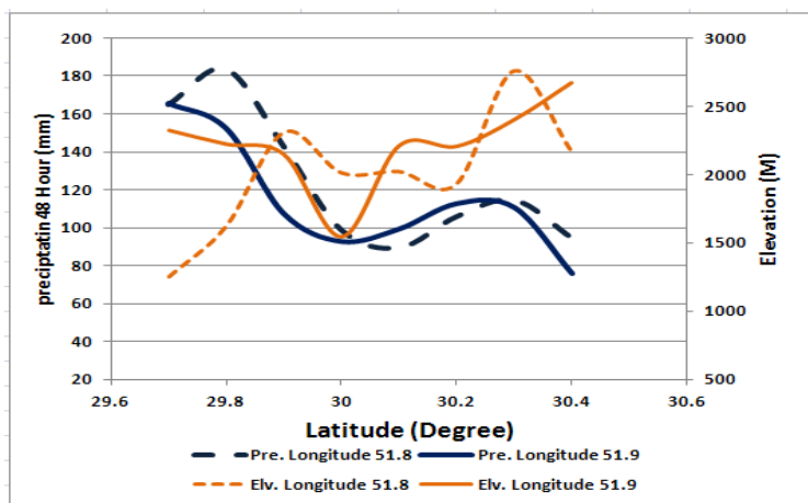
شکل (۱۲). تغییرات بارش با ارتفاع و عرض جغرافیایی در طول جغرافیایی ۵۱/۸ و ۵۱/۹ درجه توفان ۴۸ ساعته ۱۴ تا ۱۵ آذر ۱۳۸۲ در محدوده حوضه سد پارسیان
