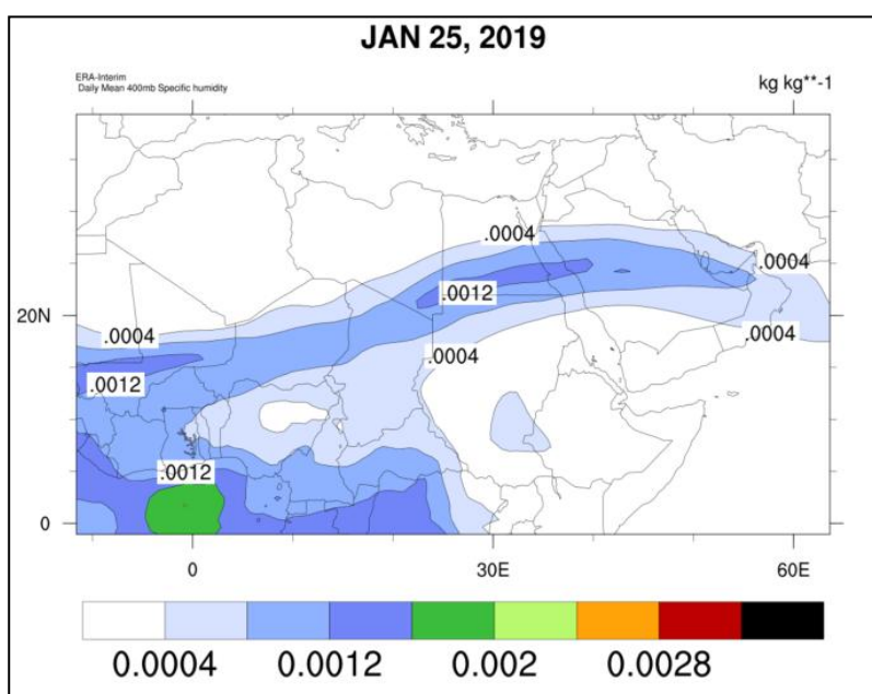
ب: رودخانه‌ی اتمسفری ۲۵ ژانویه ۲۰۱۹
