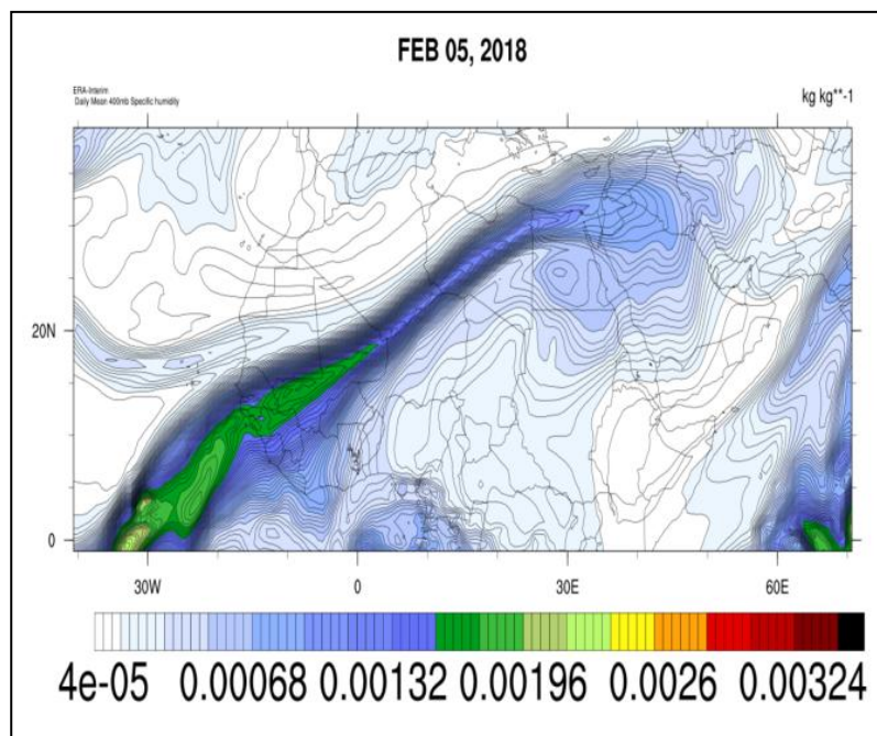
الف: رودخانه‌ی اتمسفری ۵ فوریه ۲۰۱۸
