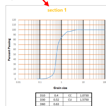
ب- منحنی دانه بندی نقطه ۱ یک، بازه مکانی یک
