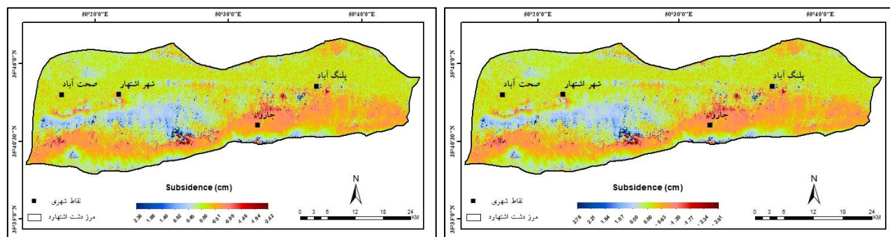
شکل (۳). فرونشست زمین در بازه زمانی (۲۰۱۸ - ۲۰۱۷)
