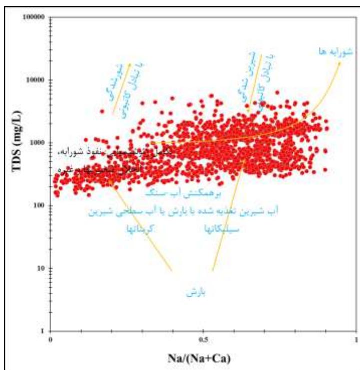
شکل (۶). موقعیت نمونه‌های مورد مطالعه بر روی دیاگرام گیبس بهینه شده
