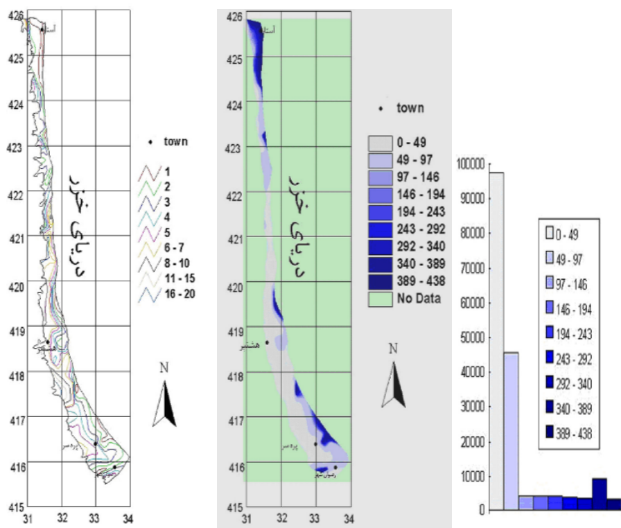
شکل ۴: هیستوگرام تبخیر آب زیرزمینی
