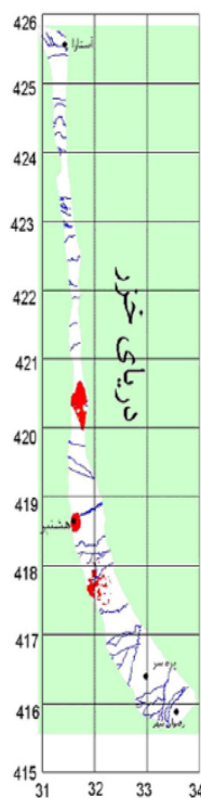
شکل ۸: مناطق مناسب جهت حفر چاه با دبی ۱۰ لیتر در ثانیه
