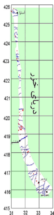
شکل ۷: مناطق مناسب حفر چاه با دبی پنج لیتر در ثانیه در
