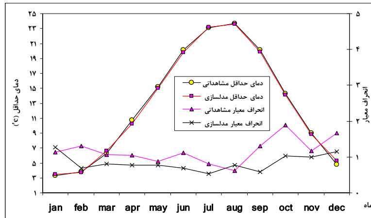
شکل (۲) نمودار میانگین ماهانه مشاهداتی و شبیه سازی شده دمای حداقل و انحراف معیار آنها در ایستگاه گرگان (۱۹۹۳-۲۰۰۷)
