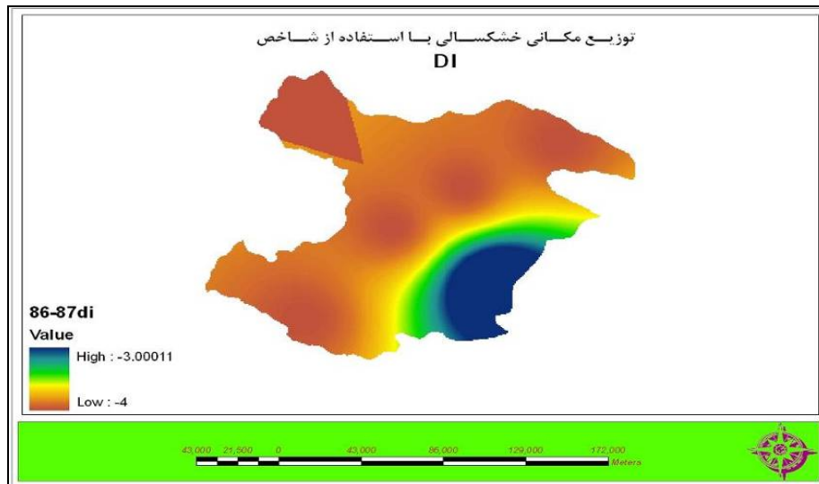
شکل (۶) توزیع مکانی خشکسالی با استفاده از شاخص DI در سال ۸۶-۸۷
