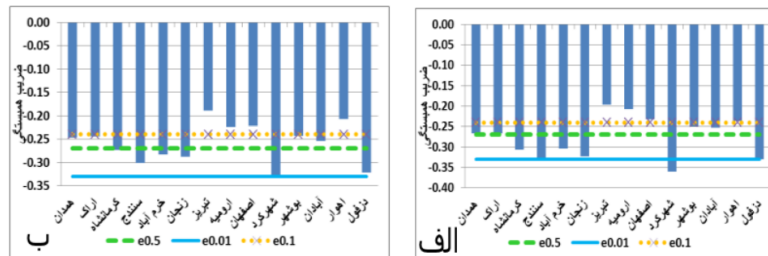
شکل (۶). مقادیر همبستگی ناهنجاری بارش ایستگاه‌های مطالعاتی با تغییرات دما تراز ۸۵۰ (الف)، دما تراز ۸۵۰ هکتوپاسکال در منطقه شرق دریای مدیترانه (ب).
