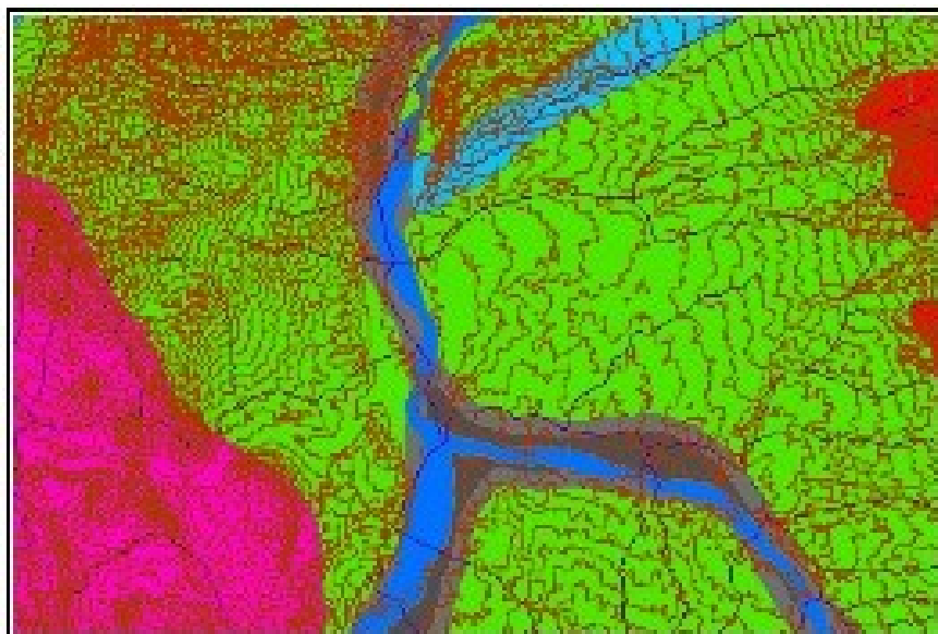
شکل (۹). تفاوت شیب زمین‌شناسی و توپوگرافیکی دو طرف چاله زنگنه
