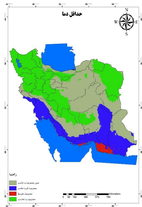
شکل (۱۳). نقشه حداکثر دما
