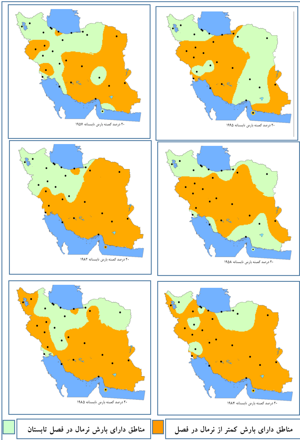
شکل (۶) پراکنندگی جغرافیایی ایستگاه‌هایی که در تابستان، طی ۳۰ ساله اول و دوم بارش شمال و کمتر از شمال
