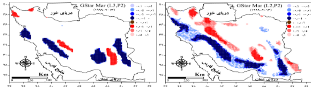
شکل (۳). نقشه‌های خودهمبستگی فضایی VIMFC زانویه تا مارس بر روی ایران طی دوره اول ۱۹۷۹-۱۹۹۸ (P1) و دوم ۲۰۱۲-۱۹۹۹ (P2). منظور از L1 لایه اول، L2 لایه دوم، L3 لایه سوم است.
