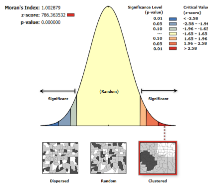
شکل (۴) الف) الگوی خوشه‌ای خشکسالی متوسط
