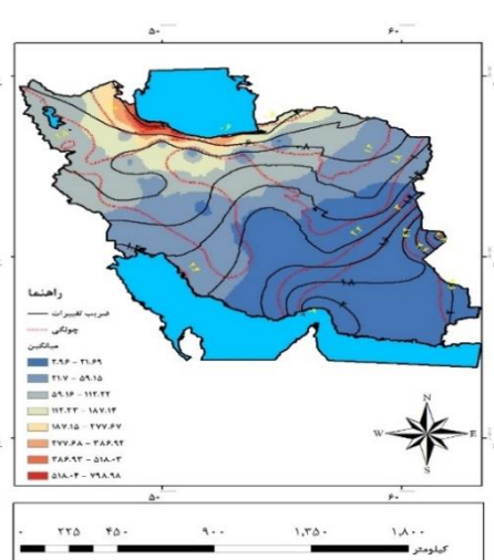
شکل (۲). میانگین، شاخص ضریب تغییرات و چولگی بارش فصل پاییز در یک دوره ۵۰ ساله (۱۹۶۱-۲۰۱۰)
