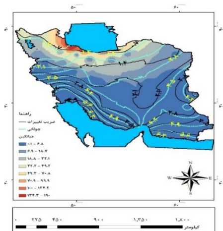
شکل (۵). میانگین، شاخص ضریب تغییرات و چولگی بارش فصل تابستان در یک دوره ۵۰ ساله (۱۹۶۱-۲۰۱۰)
