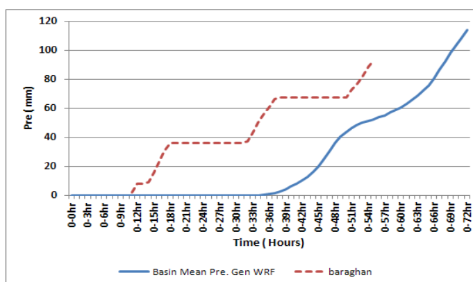
شکل (۴). مقایسه تغییرات الگوی زمانی بارش ایستگاه برغان و مدل عددی WRF (کل حوضه) بازه زمانی ۳ و ۵ دی ۱۳۸۴
