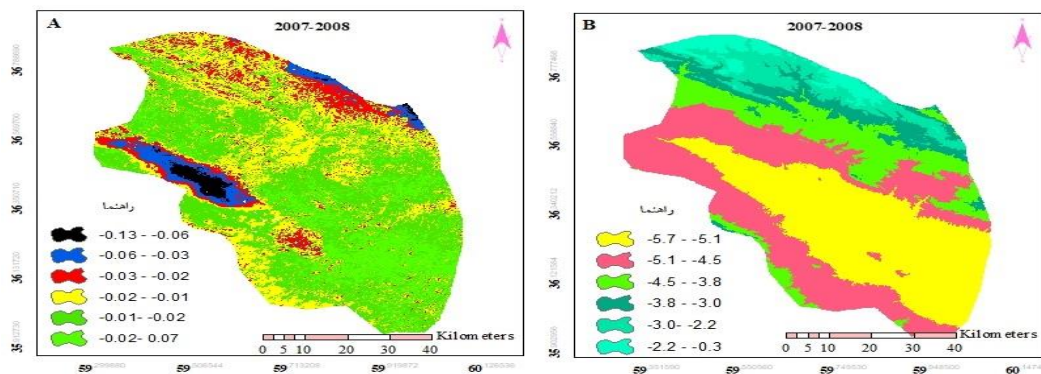
شکل (۴): (A)، دامنه فرونشست منطقه با استفاده از تصاویر سنجنده ASAR (m)، (B): درون‌یابی سطح آبهای زیرزمینی با استفاده از آمار چاه‌های پیزومتر (cm)
